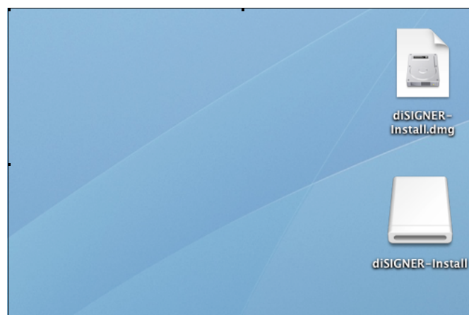
Abb. 2.2: Archiv „ diSIGNER-Install.dmg“
