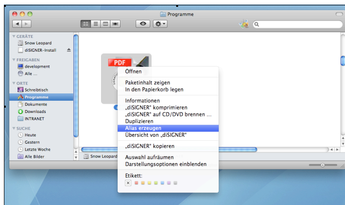
Abb. 2.4: Programm - Verzeichnis
