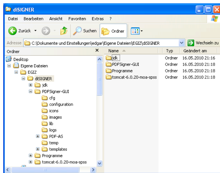
Abb. 3.2: Verzeichnis „ .../EGIZ/Programme/Mocca “
