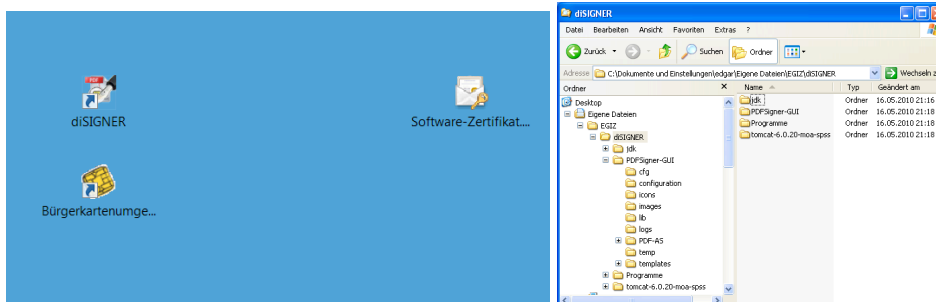
Abb. 2.12: Verzeichnis-Struktur
