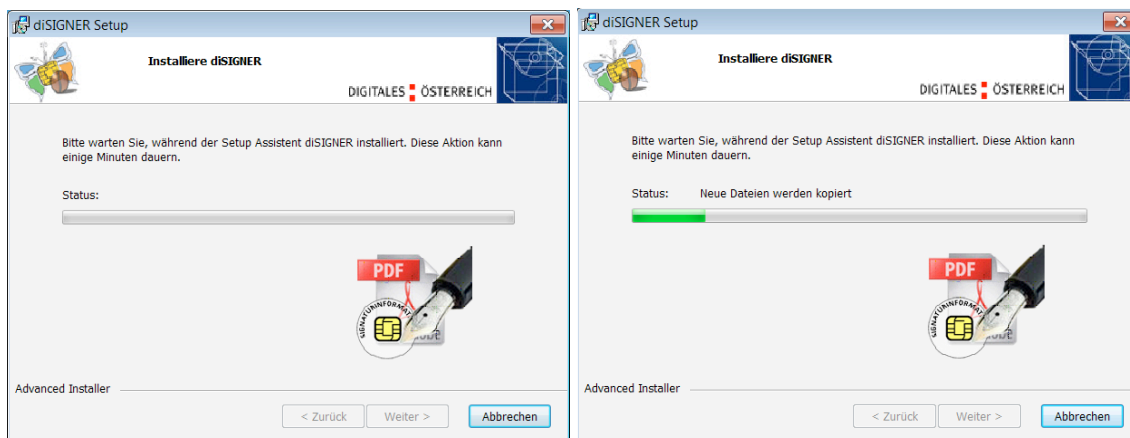
Abb. 2.8: Setup – Fortschrittsbalken
