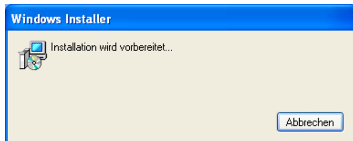
Abb. 2.2: Installation vorbereiten
